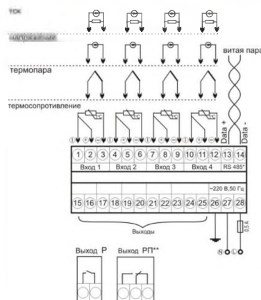
Схема расположения и состав выходов
